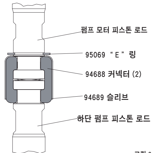
펌프 연결 세부도
